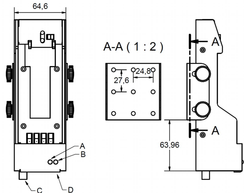
Schemazeichnung WTC1904
